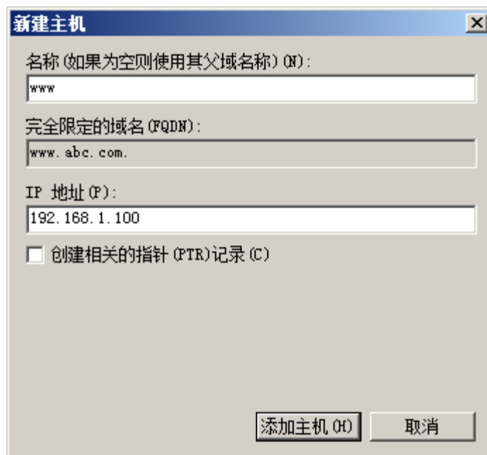
图 5 新建主机记录
