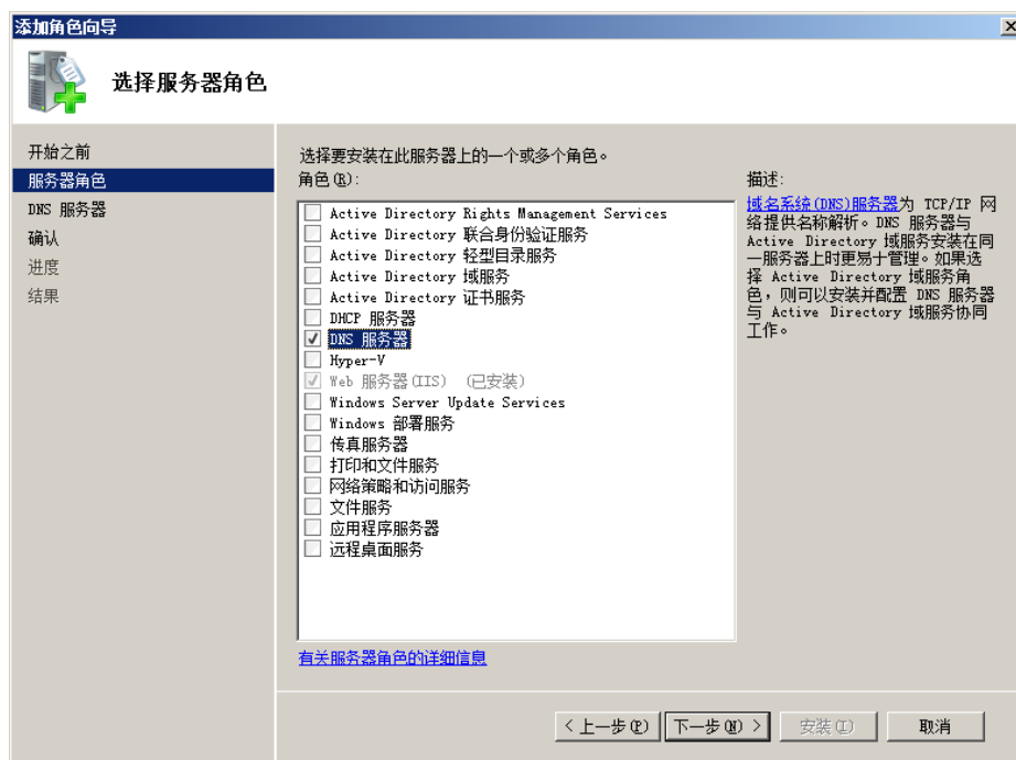
图 1 选择 DNS 服务器并安装
